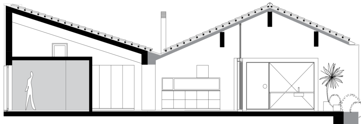
PRESJEK
